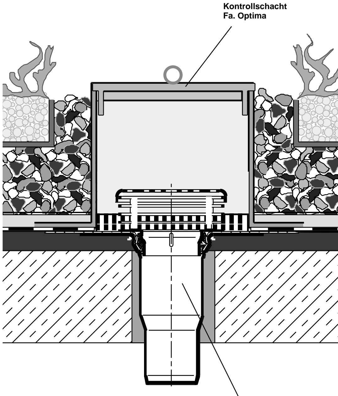
Dachablauf der Serie O Art.Nr.17110.100A
